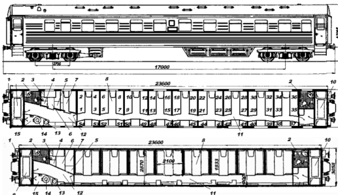
Рисунок 3.3. Пассажирский вагон
