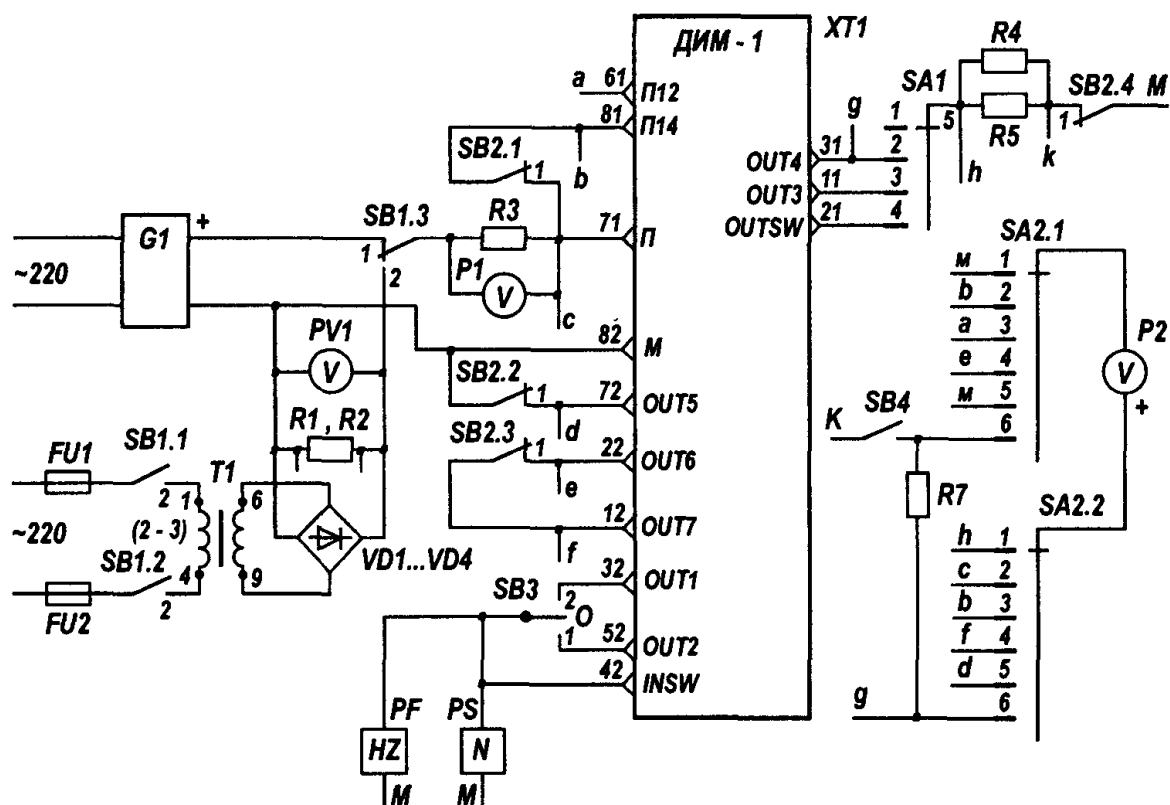
Рис. 4.24. Схема проверки датчика ДИМ-1
