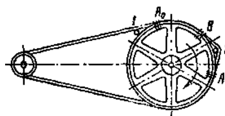
Рис. 18.4. Схема процесса укорачивания цепи. 1 и 2 – начальное и конечное положение деревянного бруса диаметром 25 – 30 мм; A_0 – места начального крепления; А и В – места конечного крепления цепи к ободу звездочки
