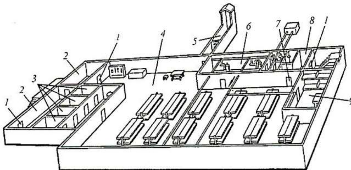
Рис.7.5. Планировка убежища
