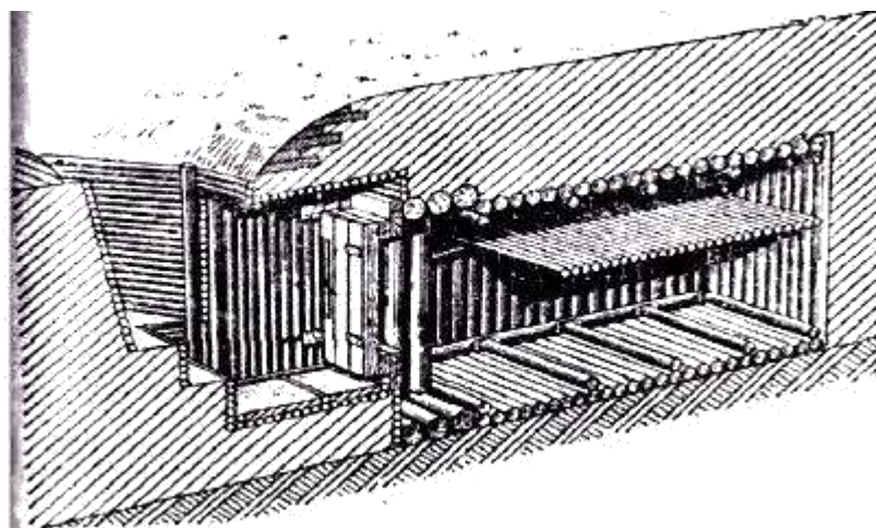
Рисунок 2.2. Блиндаж безврубочной конструкции на 6 – 8 человек
