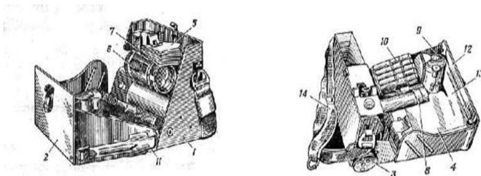
Рисунок 3.3. ВПХР: 1 — корпус; 2 — крышка; 3 — ручной насос; 4 — кассеты с индикаторными трубками; 5 — противозарозольные фильтры; 6 — насадка; 7 — защитные колпачки; 8 — фонарь; 9 — грелка; 10 — патроны к грелке; 11 — лопатка; 12 — инструкция-памятка по работе с прибором; 13 — инструкция по обнаружению фосфорорганических ОВ; 14 — плечевой ремень.
